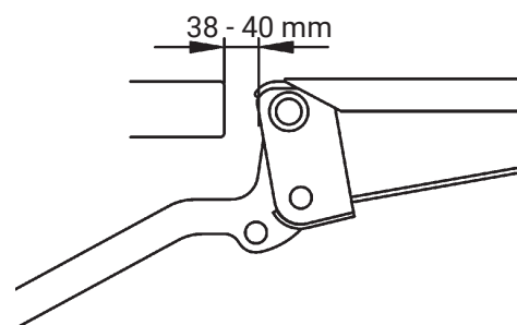
Abbildung 30. Sicherstellen, dass der Abstand zwischen Ladefläche und Bordwand 38–40 mm beträgt
