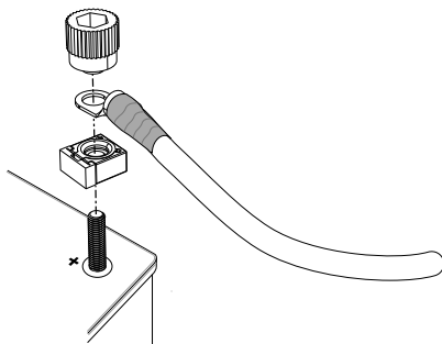
Abbildung 55. Anschließen an den Pluspol der Batterie
