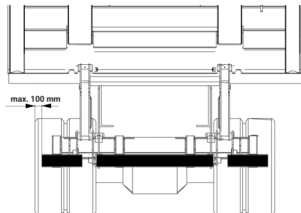
Abbildung 10. Gesetzlich vorgeschriebene Maße
