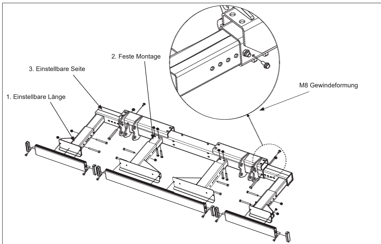
Abbildung 41. Montage Unterfahrschutz
