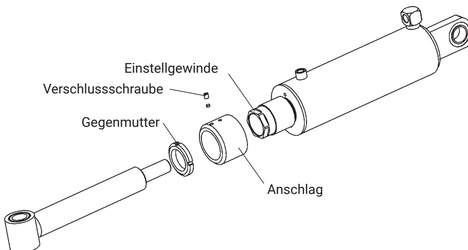
Abbildung 40. Den Anschlag ausrichten
