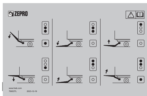
Abbildung 76. Steuergeräteaufkleber für CD1 mit Zweihandtaster unterhalb des Steuergerätes montiert.
