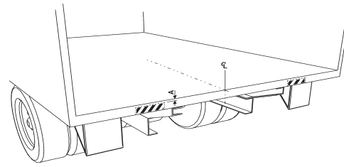
Abbildung 17. Mittelpunkt an der Hecktraverse ausmessen und markieren
