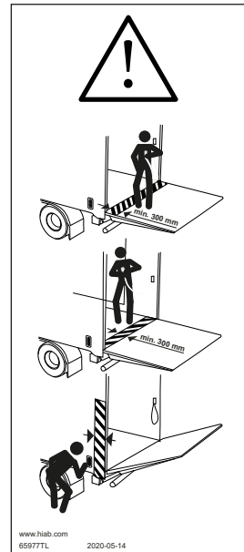
Abbildung 78. Gefahrenbereich
