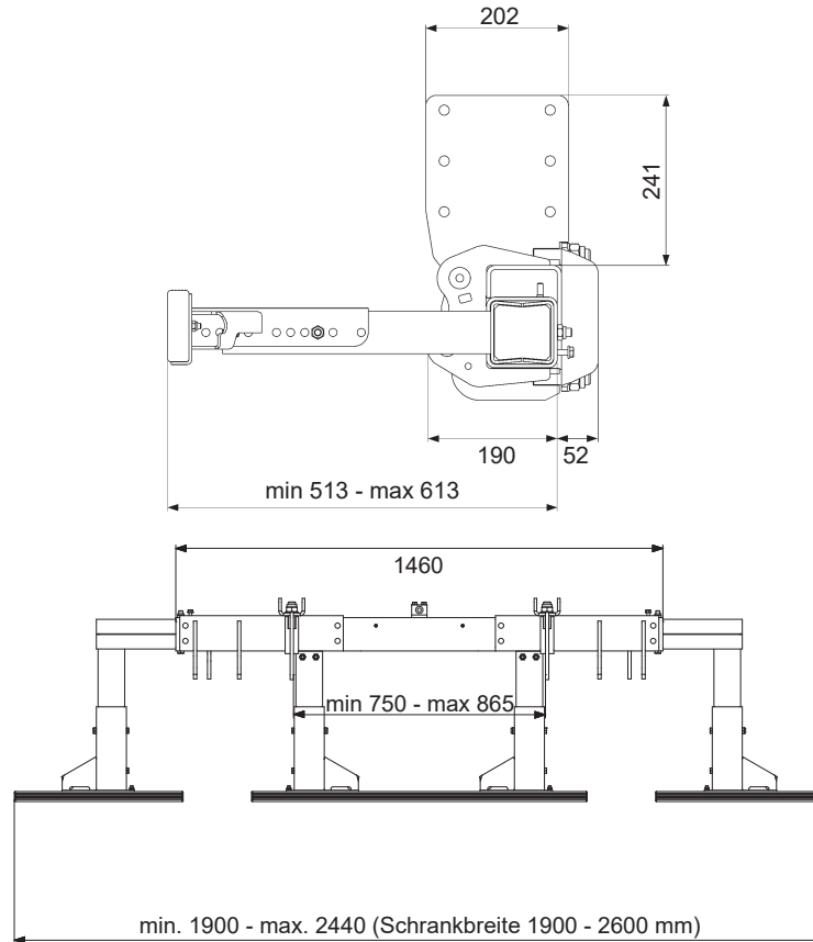
Abbildung 12. Z-100-110
