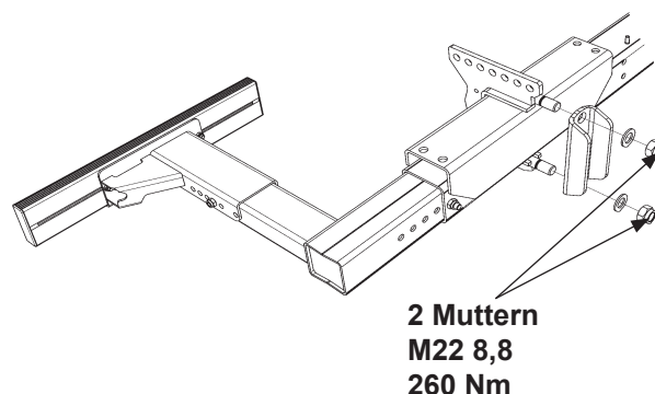
Abbildung 20. Rahmenhalter montieren
