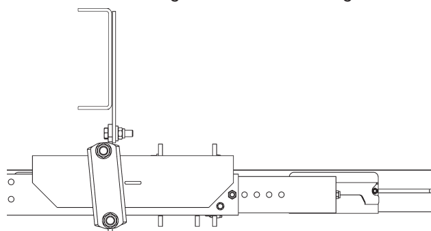
Abbildung 23. Montage die Rahmenhalter, wenn die Breite des Fahrzeugrahmens größer als 960 mm beträgt
