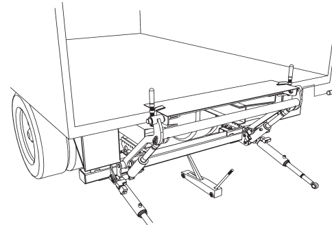
Abbildung 19. Justieren Sie die Aufhängung bis zur Idealhöhe unter dem Rahmen
