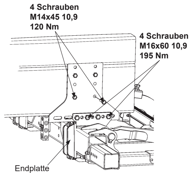
Abbildung 24. Montage des Hubträgers
