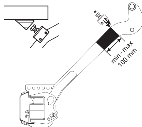
Abbildung 32. Armanschlag montieren
