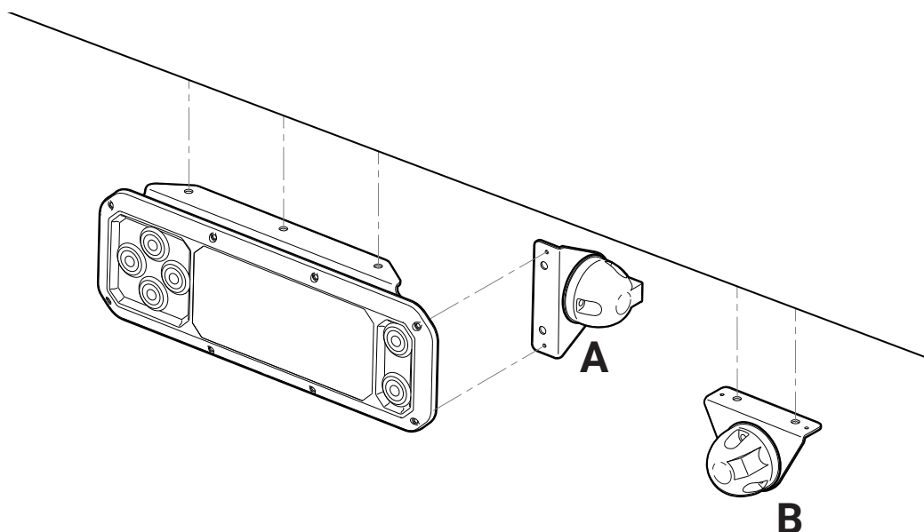
Abbildung 51. Montage der Bedienvorrichtung CD19 und des Anschlusses für die Handbedienung
