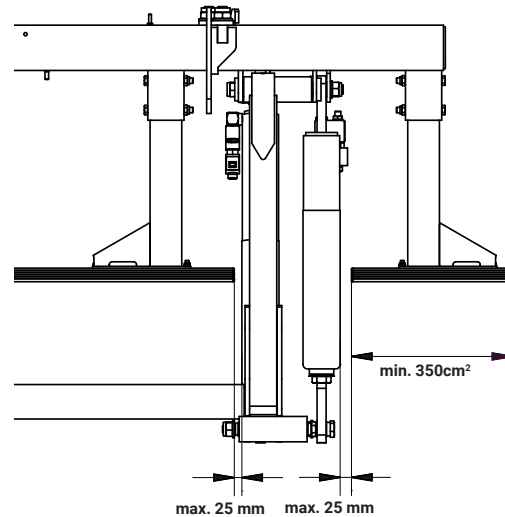
Abbildung 9. Gesetzlich vorgeschriebene Maße
