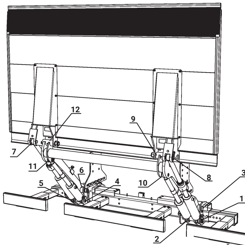
Abbildung 64. Schmierpunkte
