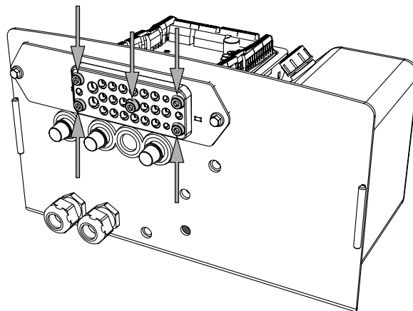
Abbildung 58. Die fünf Schrauben der Kabeldurchführung
