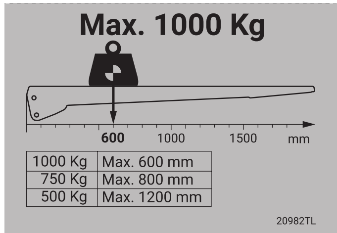
Abbildung 66. Lastdiagramm für eine Tragfähigkeit von 1000 kg, Schwerpunktabstand 600 mm
