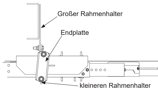
Abbildung 22. Montage die Rahmenhalter, wenn die Breite des Fahrzeugrahmens weniger als 770 mm beträgt
