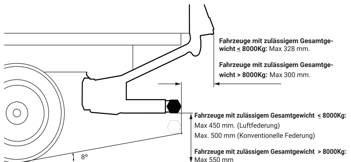
Abbildung 8. Gesetzlich vorgeschriebene Maße
