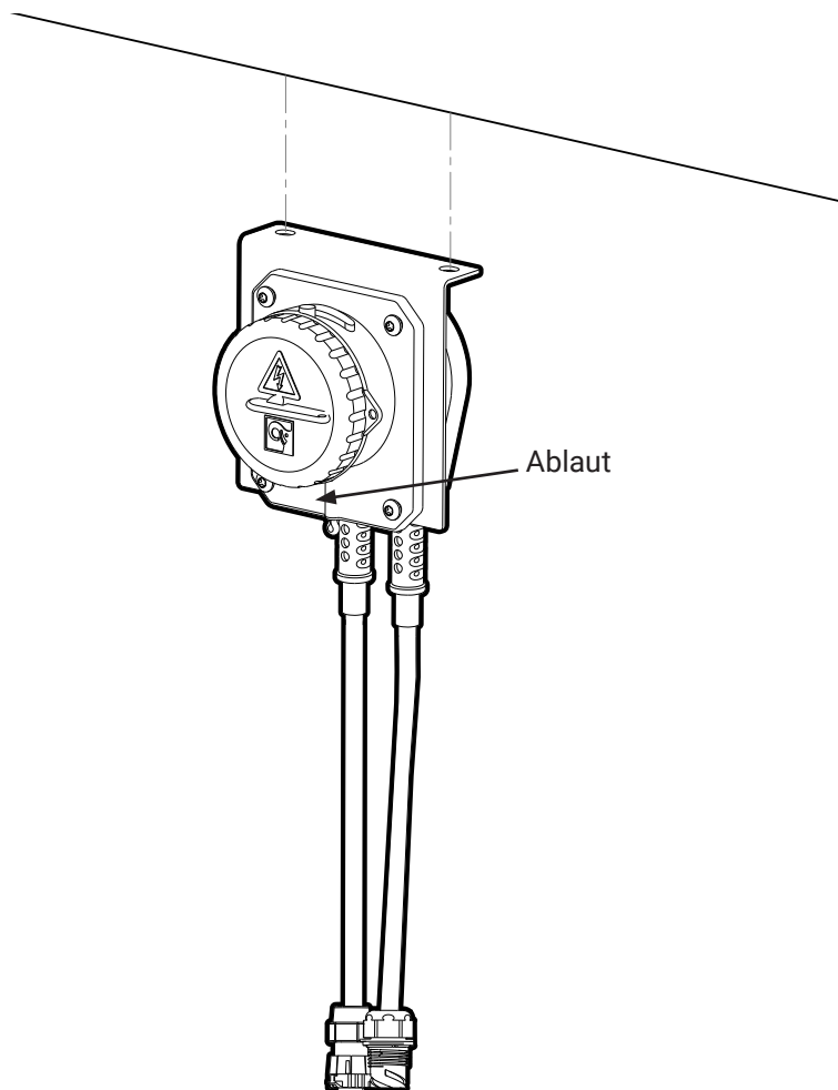
Abbildung 57. Montage des Hauptschalters
