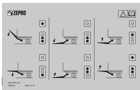
Abbildung 75. Steuergeräteaufkleber für CD 1 mit oberhalb des Steuergerätes angebrachtem Zweihandtaster.
