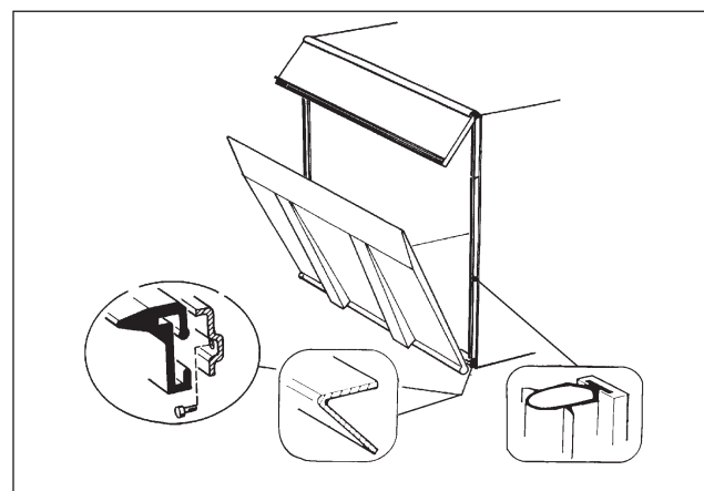
Abbildung 31. Bordwand kontrollieren
