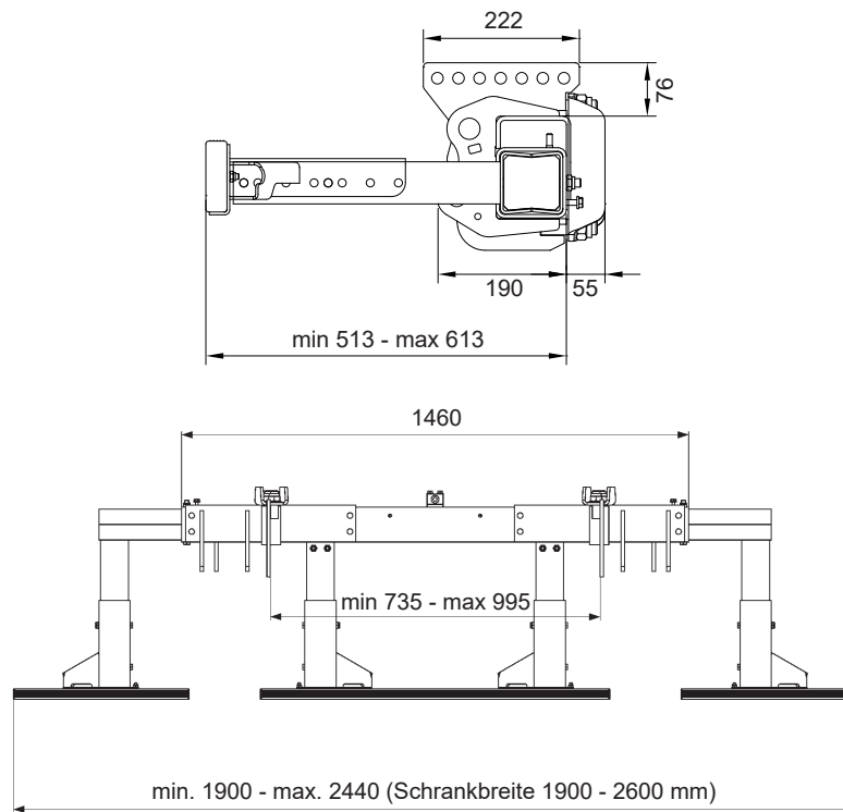
Abbildung 13. Z-100-130
