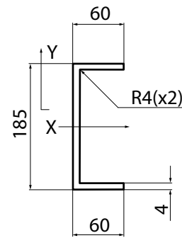
Abbildung 7. Querschnitt des betreffenden Trägers
