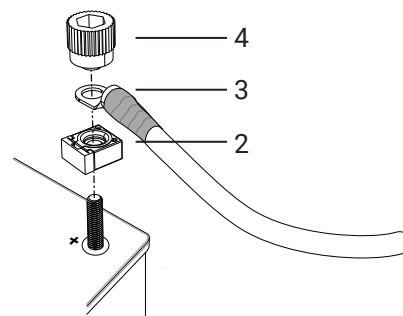
Abbildung 60. Anschließen an den Pluspol der Batterie
