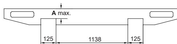
Abbildung 14. Z 100-110/130
