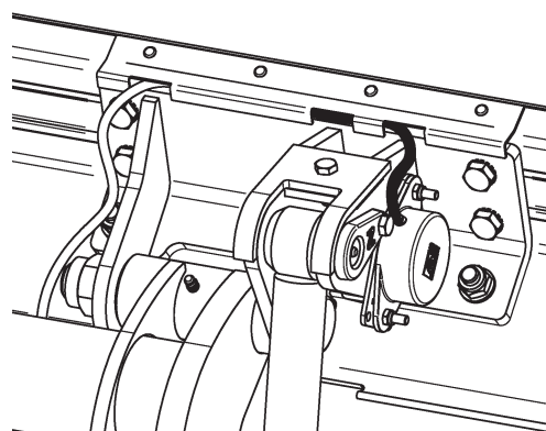
Abbildung 28. Montieren Sie die Ladebordwand an den Armen
