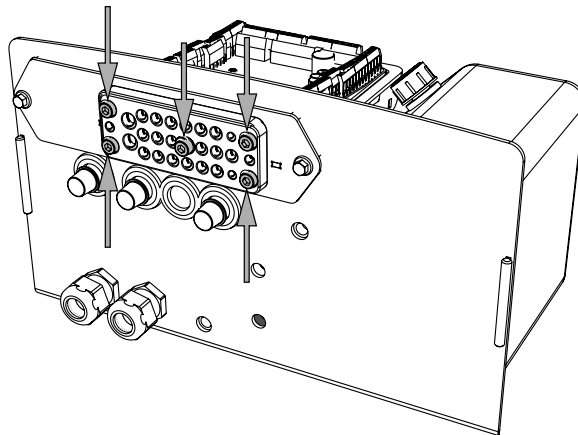
Abbildung 15. Die fünf Schrauben der Kabeldurchführung
