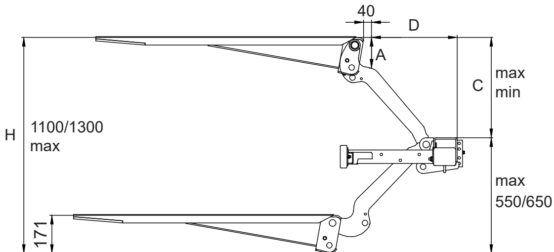
Hubhöhe 1100 mm
