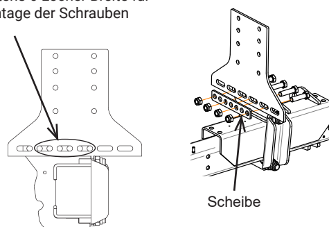
Abbildung 21. Rahmenhalter montieren
