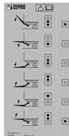
Abbildung 72. Bedienungsaufkleber für CD 1, 2, 9
