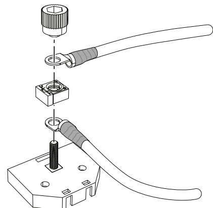
Abbildung 56. Anschließen an den Sicherungskasten
