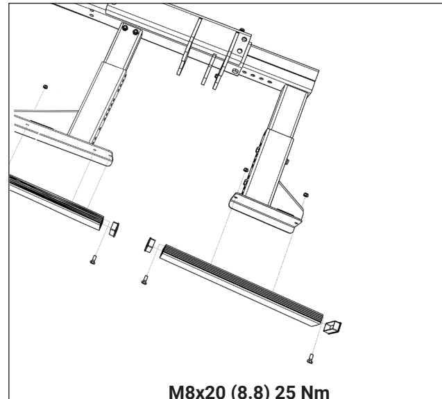
Abbildung 42. Befestigen Sie die Aluminiumprofile mit je 2 Bolzen M8x20 (8,8) und ziehen Sie diese mit dem Anzugsdrehmoment 25 Nm fest
