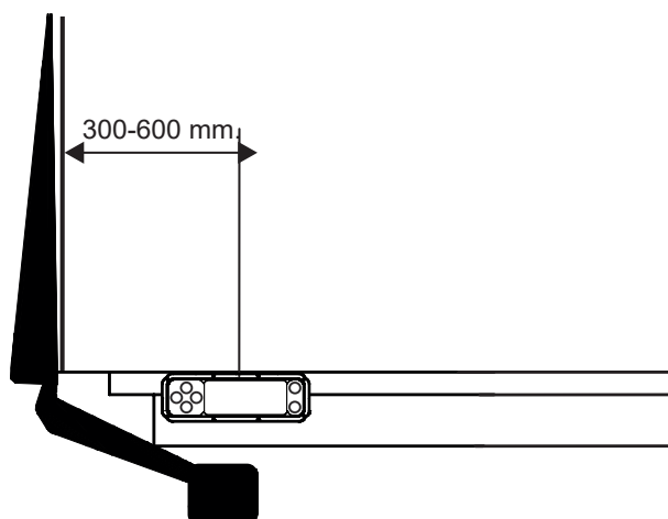
Abbildung 44. Montage der Bedienvorrichtung
