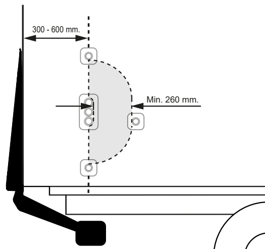
Figure 61. Installation de l'actionneur CD 1 pour une utilisation à deux mains.
