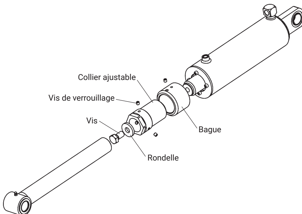
Figure 46. Vérin d'inclinaison
