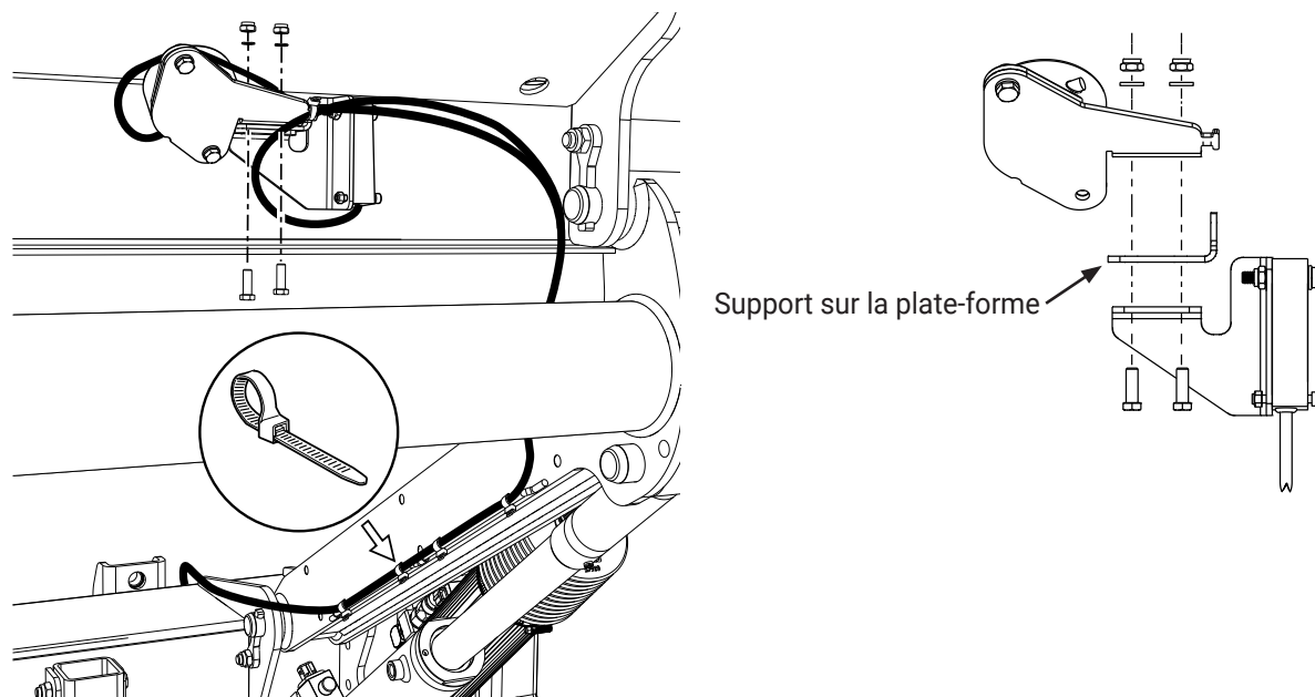
Figure 58. Capteur d'angle de montage pour ouverture / fermeture automatique
