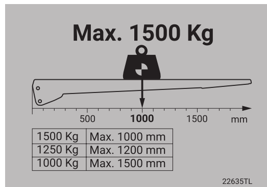
Figure 88. Le diagramme de charge pour la capacité de charge 1500 kg, distance du centre de gravité 1000 mm.
