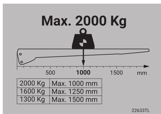
Figure 89. Le diagramme de charge pour la capacité de charge 2000 kg, distance du centre de gravité 1000 mm.
