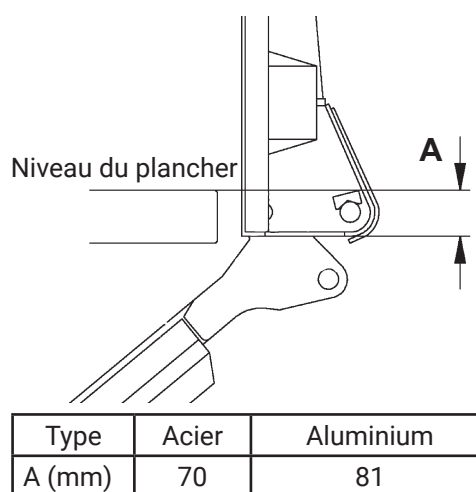
Figure 37. Le porte-à-faux (A) de la plate-forme varie selon les différents types de ponts, ce qui doit être pris en compte lors de l'installation d'une bande d'étanchéité sur le bord supérieur.
