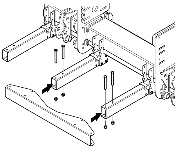
Figure 53. Installation d'un profil en tôle intérieur
