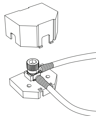
Figure 85. Boîte à fusibles avec couvercle de protection
