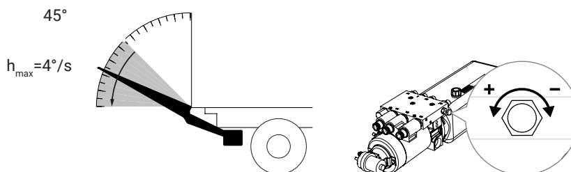
Figure 55. Réglage de la vitesse de givrage vers le bas dans la plage de travail (à partir de 45° vers le bas)
