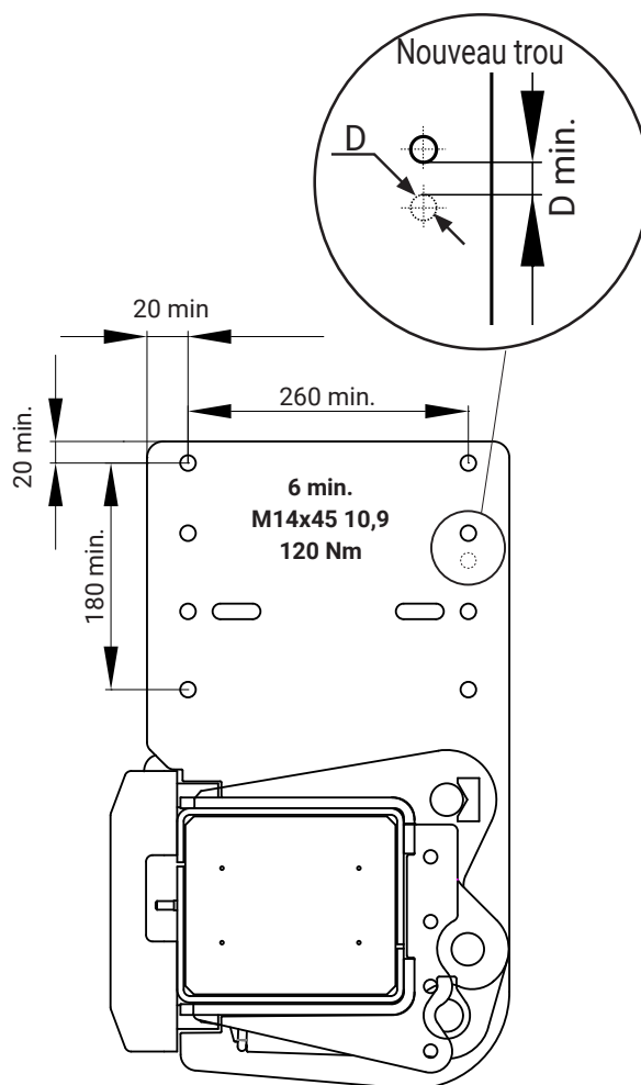
Figure 31. Fixation du support de cadre avec au moins 6 vis M14x45 10,9
