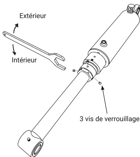
Figure 38. Réglage de l'angle d'inclinaison
