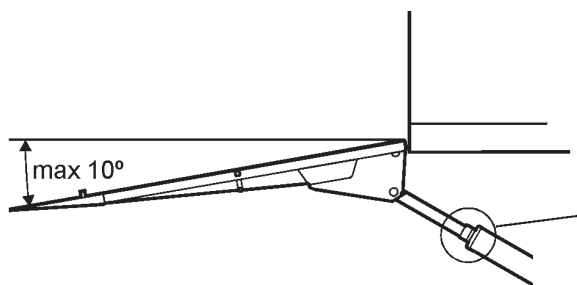
Figure 44. Ajustement de l'angle d'inclinaison basse à 10° max.
