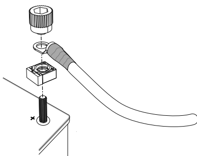
Figure 71. Connexion au pôle plus de la batterie
