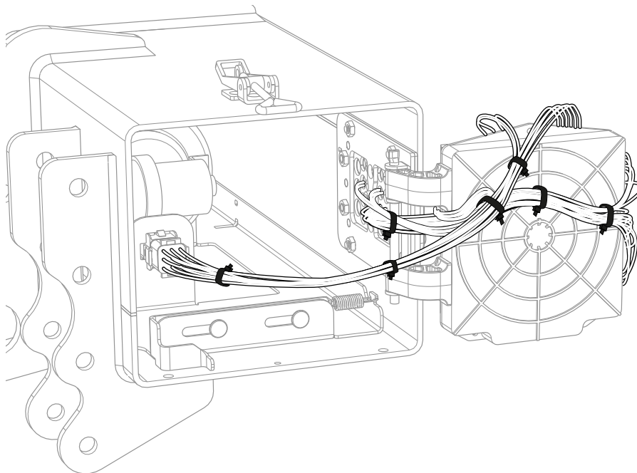
Figure 80. Mise en place des faisceaux avec serre-câbles
