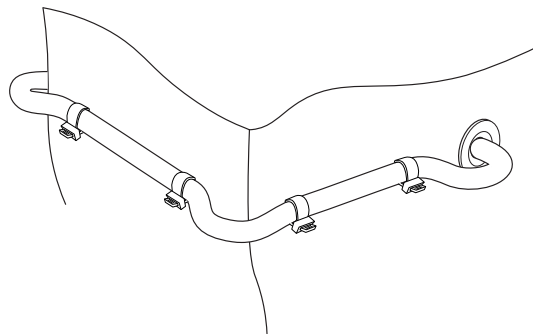
Figure 68. Protégez le câble de toute arête vive et utilisez des presse-étoupes
