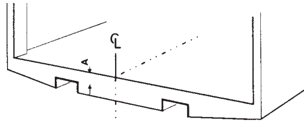
Figure 26. Mesurez et marquez le centre de la traverse arrière du véhicule
