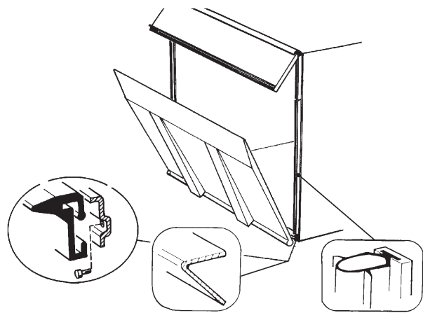
Figure 48. Pose de la bande d'étanchéité
