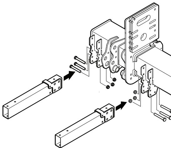
Figure 52. Montage des supports sur le tube porteur
