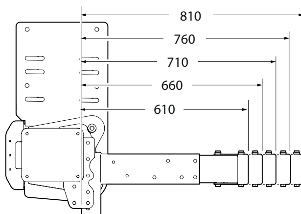
Figure 50. La partie extérieure des supports peut être montée dans cinq positions différentes
