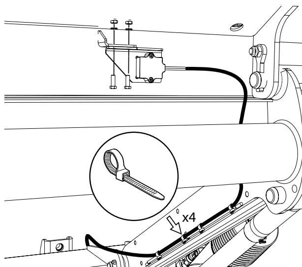
Figure 57. Montage de l'inclinomètre
