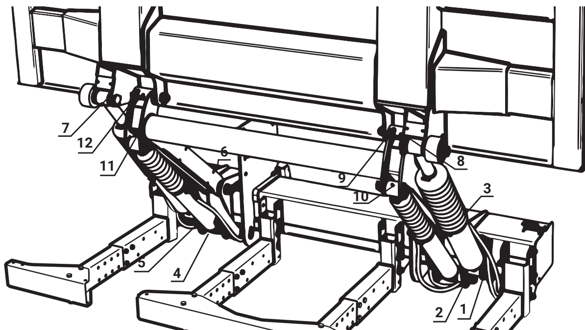
Figure 86. Points de graissage
