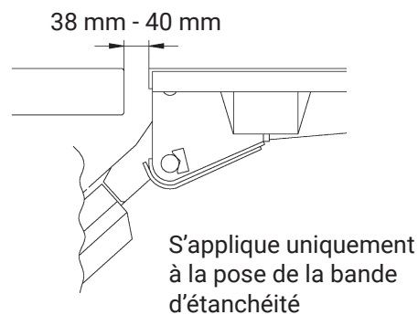
Figure 36. Contrôle de la position par rapport à la traverse arrière du véhicule
