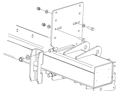
Figure 29. Fixation du profilé en U avec ses rondelles et écrous
