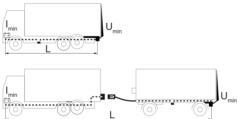
Figure 70. Capacité de la batterie et définition de la longueur du câble d'alimentation principal et de terre
