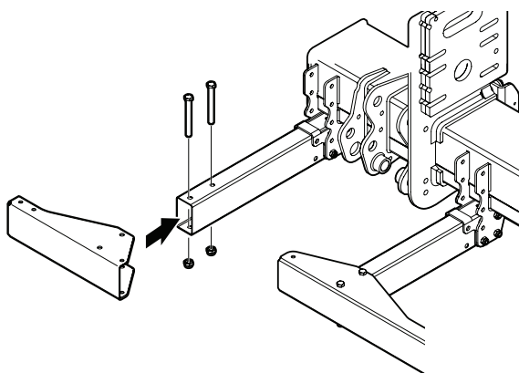
Figure 53. Installation d'un profil en tôle intérieur
