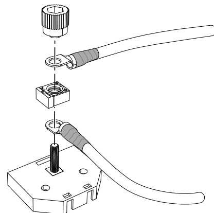
Figure 72. Connexion à la boîte à fusibles
