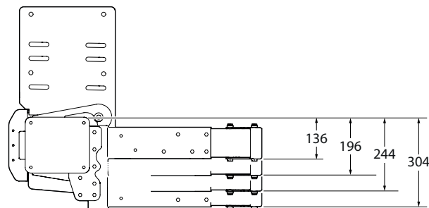
Figure 49. La partie intérieure des supports peut être montée à quatre hauteurs différentes
