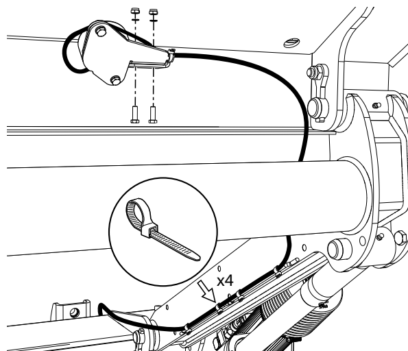
Figure 56. Montage du capteur angulaire
