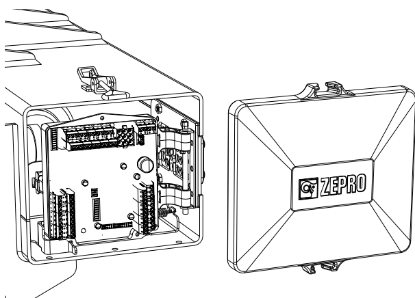
Figure 19. Démontez le capuchon de protection
