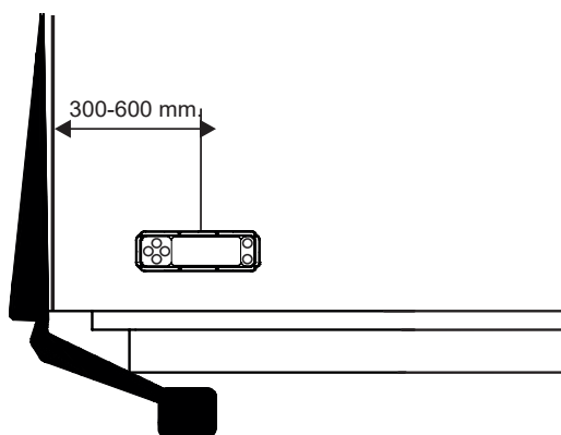
Figure 63. Installation de l'actionneur
