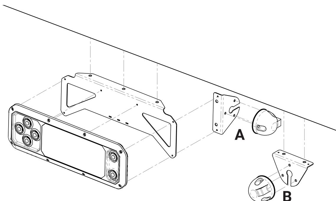
Figure 67. Montage de l'actionneur portable CD 19 et contact pour l'actionneur portable
