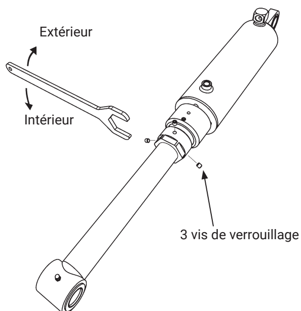
Figure 40. Réglage de l'angle d'inclinaison
