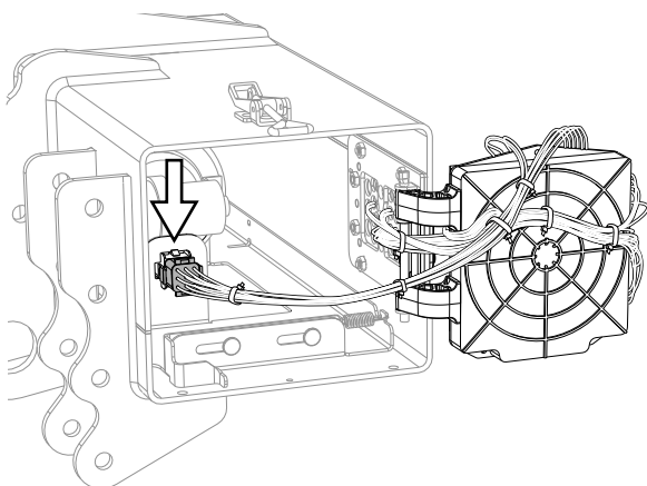
Figure 21. Connecteur
